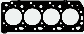
TC-326-07 - 1005A205/06 Junta Culata de Cilindros Junta Cabeçote
