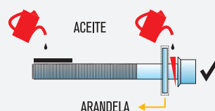
TORNILLO DE CULATA CON ARANDELA
