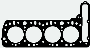
TC-775-20 - 6160162020 6210100321/100009500 Junta Culata de Cilindros Junta Cabeçote
