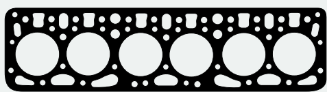
TC-325-20 - 3210160220 Junta Culata de Cilindros Junta Cabeçote
