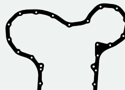
1090700 - 287553 Tapa distribución Tampa distribuição
