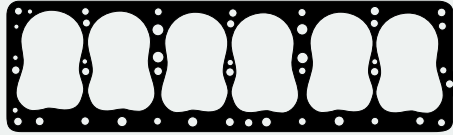
TC-190-05 Junta Culata de Cilindros Junta Cabeçote
