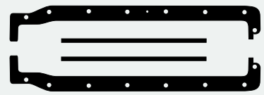
JC-275-26 Junta Carter Junta Carter
