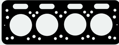
TC-220-02 - 8807696 Junta Culata de Cilindros Junta Cabeçote
