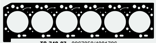
TC-740-07 - 3967059/4981796 Junta Culata de Cilindros Junta Cabeçote
