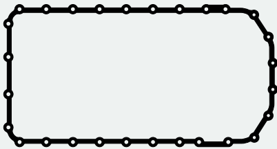
JC-392-25 - R521525 Junta Cáster (agujeros 11mm) Junta Carter (furos 11mm)
