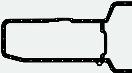
JC-152-34 - 573228 Junta Cártel Junta Carter
