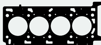
TC-959-11 - 8200805657 Junta Culata de Cilindros Junta Cabeçote
