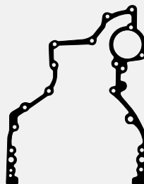
1178600 - 836647419 Tapa distribución Tampa distribuição
