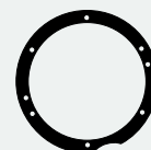
1097600 - 22020143 Suplemento bancada trasera Suplemento mancal traseira (0,40mm)
