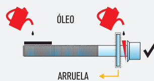
PARAFUSO DE CABEÇOTE COM ARRUELA
