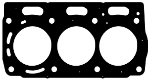
TC-707-11 3681E045/3681E049/4225270M1 Junta Culata de Cilindros Junta Cabeçote
