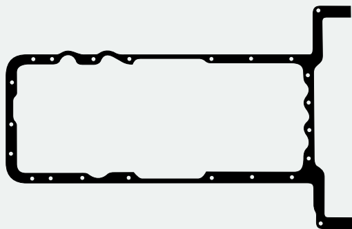
JC-288-25 Junta Cártel Junta Carter
