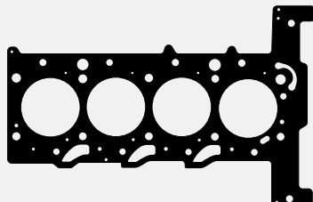
TC-891-11 - 0209EH/6C1Q6051AB Junta Culata de Cilindros Junta Cabeçote
